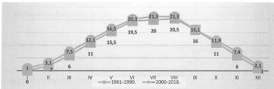
Дијаграм 6-2: Поређење средње температуре на подручју општине Нови Град за периоде 1961.-1990. и 2001.-2018.
