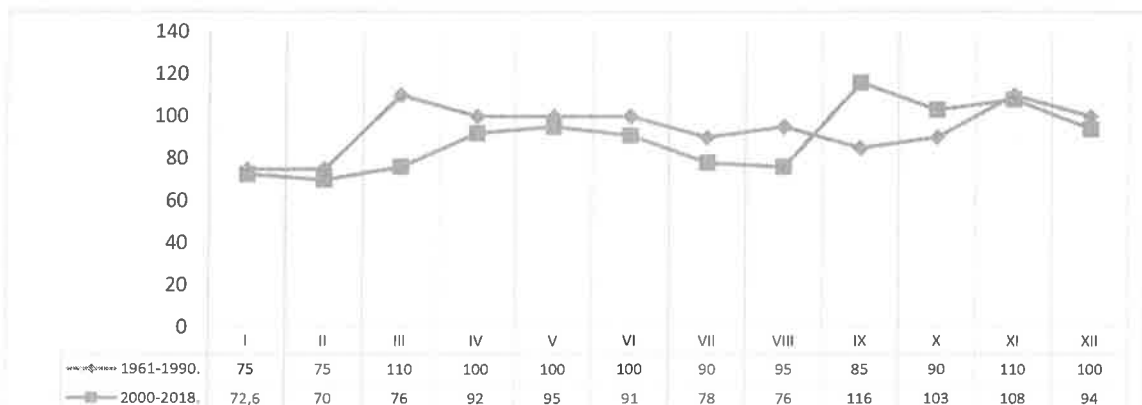
Дијаграм б-4. Поређење количине падавина за подручје општине Нови Град за периоде 1961.-1990. и 2000.-2018.
